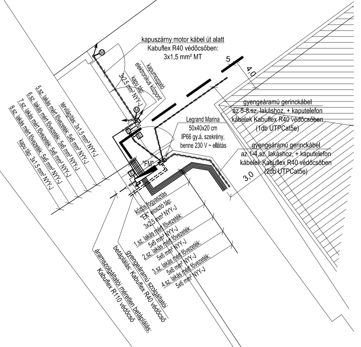
A részletrajz M 1:100
